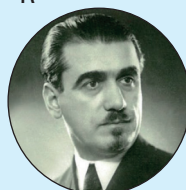
Ion
